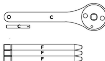
C T10195 Herramienta de bloqueo del cigüeñal 23270-03 F T10200 Juego de pasadores guía (3) 23270-06
